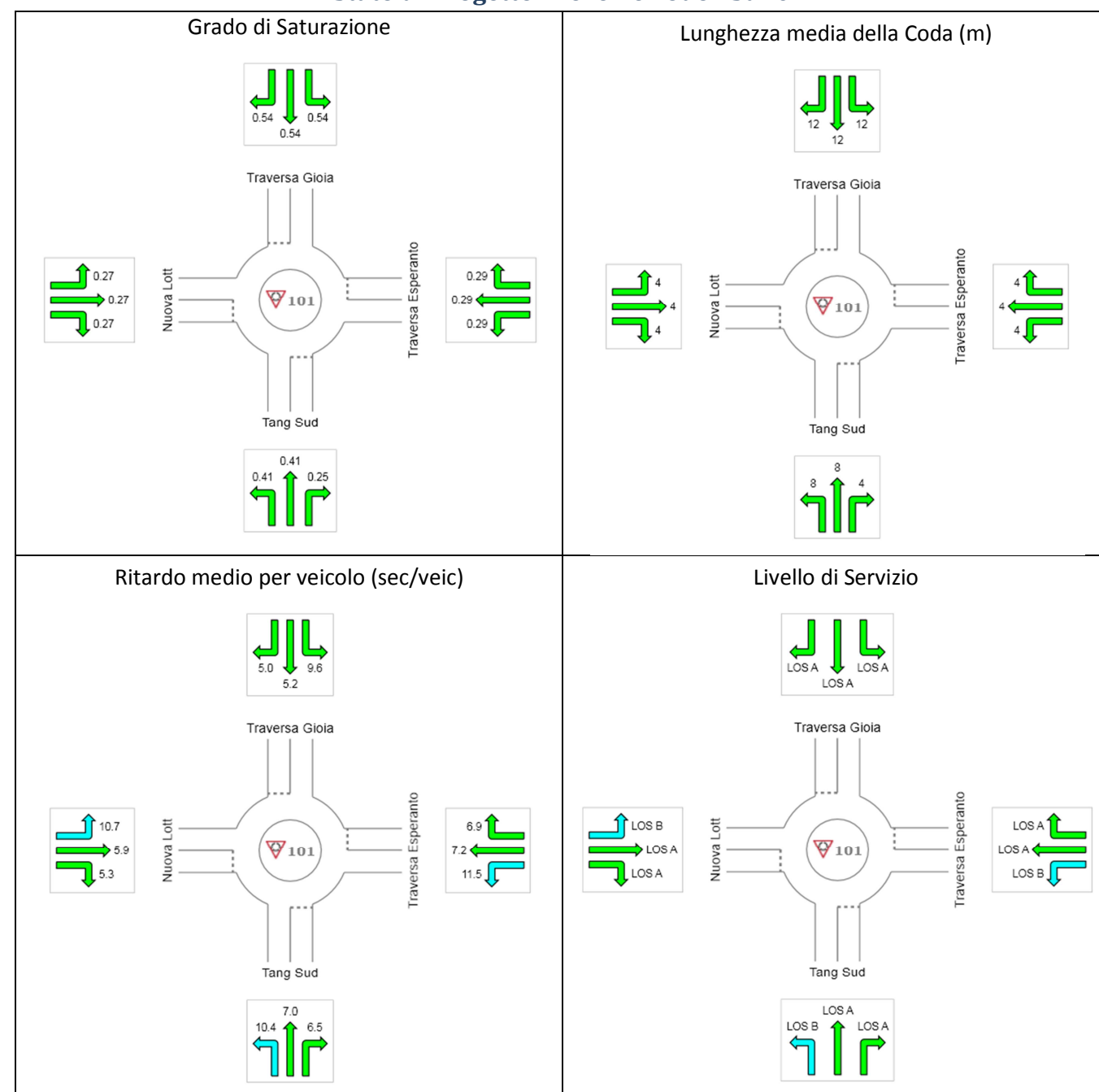
Figura 8-22: Nodo Traversa Gioia – Traversa Esperanto – Svincolo Tang Sud Risultati delle verifiche di capacità - Ora di Punta Venerdì 17.00-18.00 – SdP0
