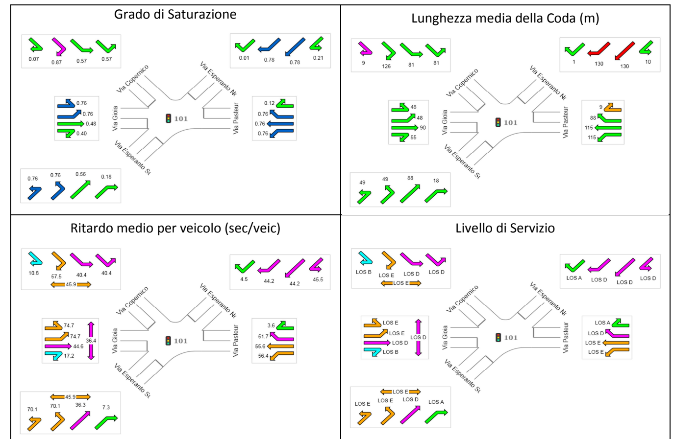
Figura 8-4: Nodo via Pasteur – via dell'Esperanto – via Copernico – via Gioia Risultati delle verifiche di capacità - Ora di Punta Venerdì 17.00-18.00 – SdF
