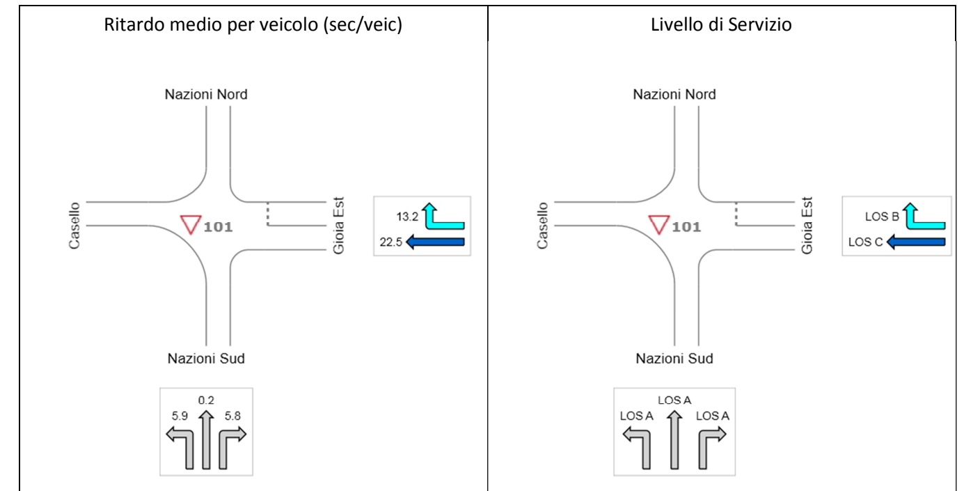
Figura 8-18: Nodo Via Gioia – Viale Nazioni – Via Fermi Risultati delle verifiche di capacità - Ora di Punta Venerdì 17.00-18.00 – SdP0
